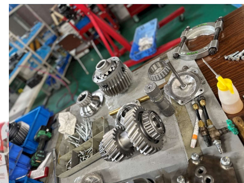
↑レース車600シリーズのトランスファーの組み立て。 納得いくまで調整を繰り返し、最高の一品を仕立てます。
